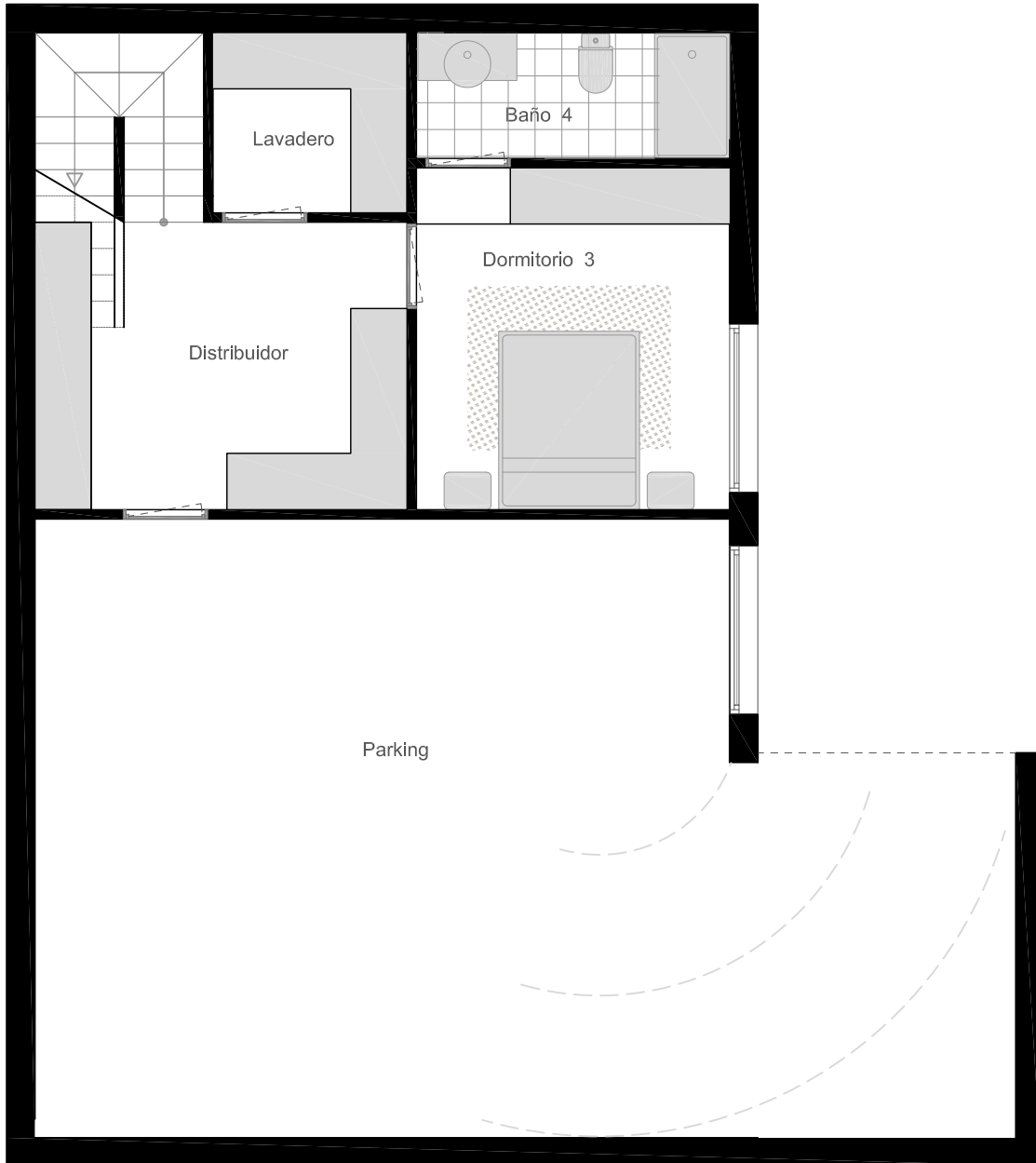
Planta sótano
