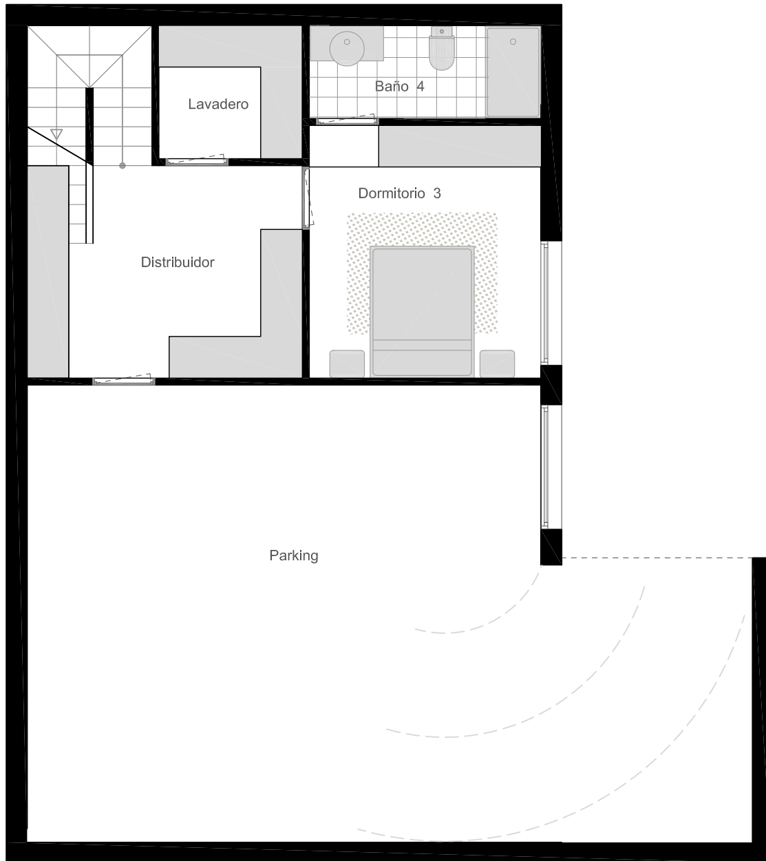
Planta sótano
