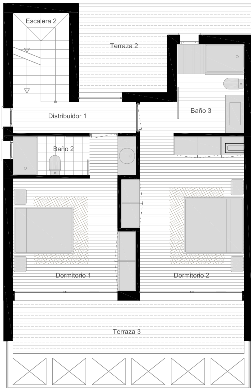
Planta primera
